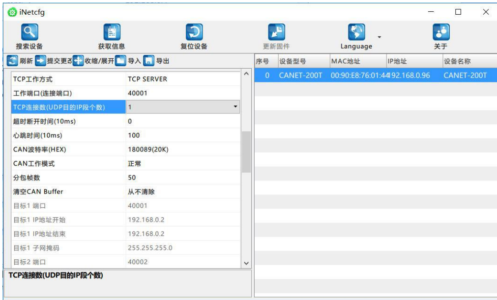
图 4.14 CAN2 配置信息
