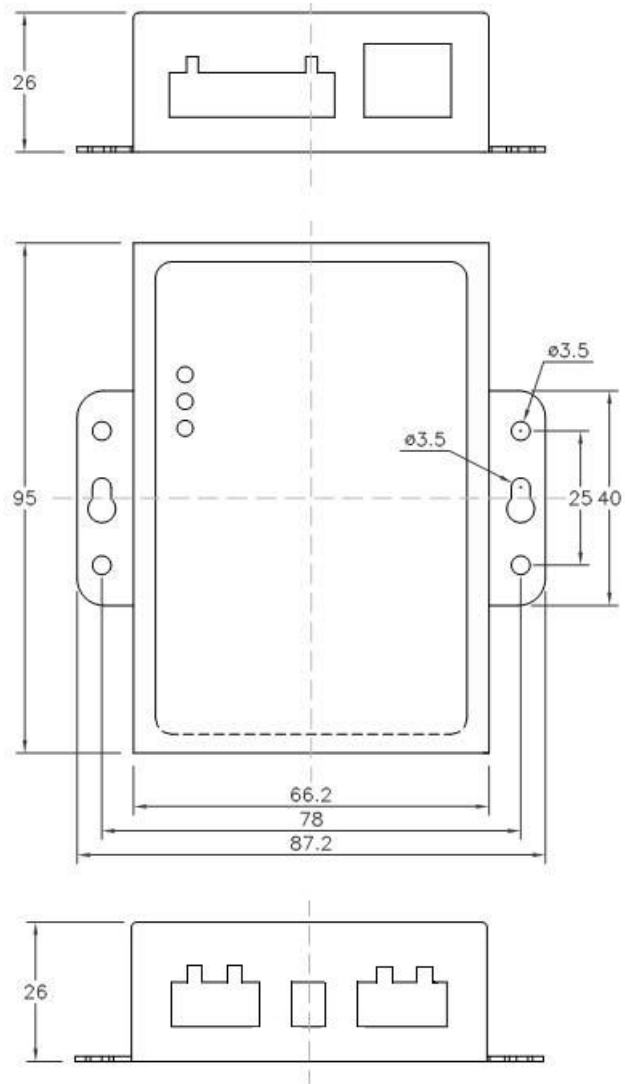
图 1.2 CANET-200T 安装机械尺寸
